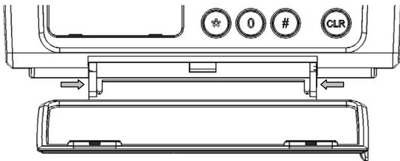
Рис. 4. Снятие крышки ПЦН
