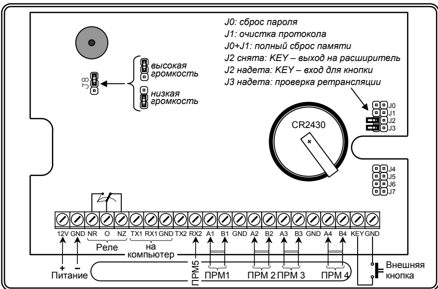
Рис. 3. Монтажная схема ПЦН
