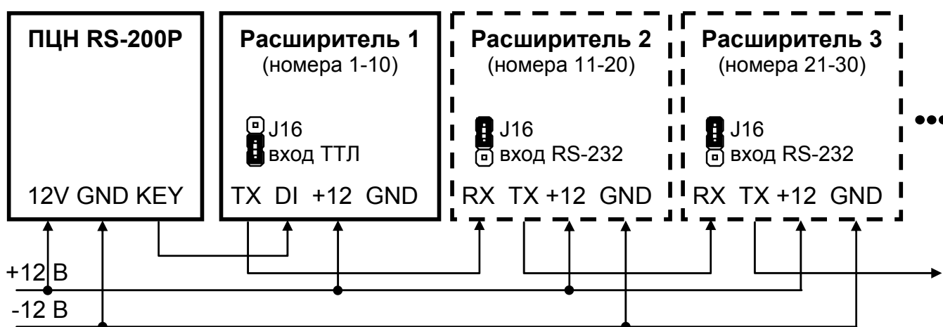
Рис. 3. Подключение расширителя к ПЦН RS-200P (до 16 шт.)
